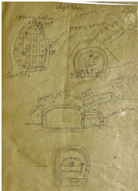
Рис. 6. Аркуш зі схематичним кресленням гончарного горна (Документи ... 1932, арк. 292).
