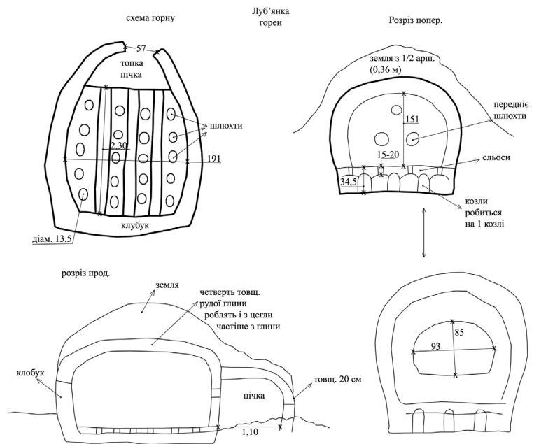
Рис. 7. Авторська промальовка креслення горна. У підписах збережено орфографію оригінального документу. До розміру, вказаного в аршинах, додано його відповідник в метричній системі (Документи ... 1932, арк. 292).
