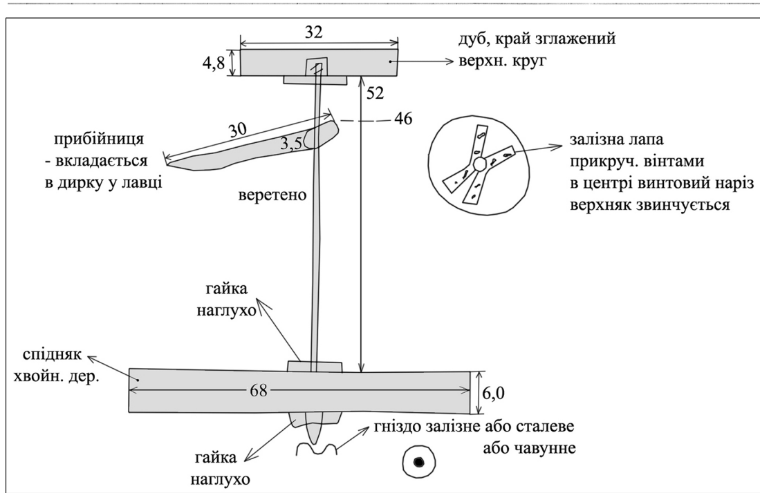
Рис. 5. Авторська промальовка креслення гончарного круга. У підписах збережено орфографію оригіналу (Документи ... 1932, арк. 290).
